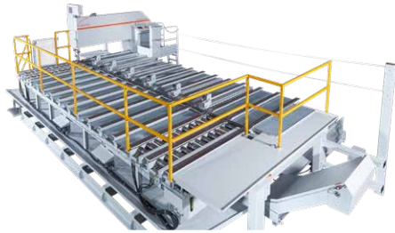
Blockbandsäge – KASTObbs A 3x20
